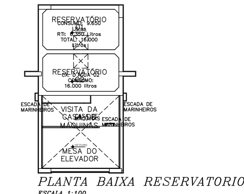
PLANTA BAIXA RESERVATÓRIO ESCALA 1:100
