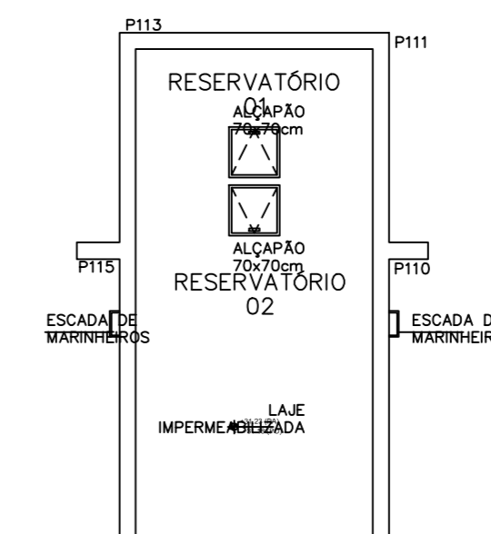
PLANTA BAIXA CX. D'AGUA ESCALA 1:100
