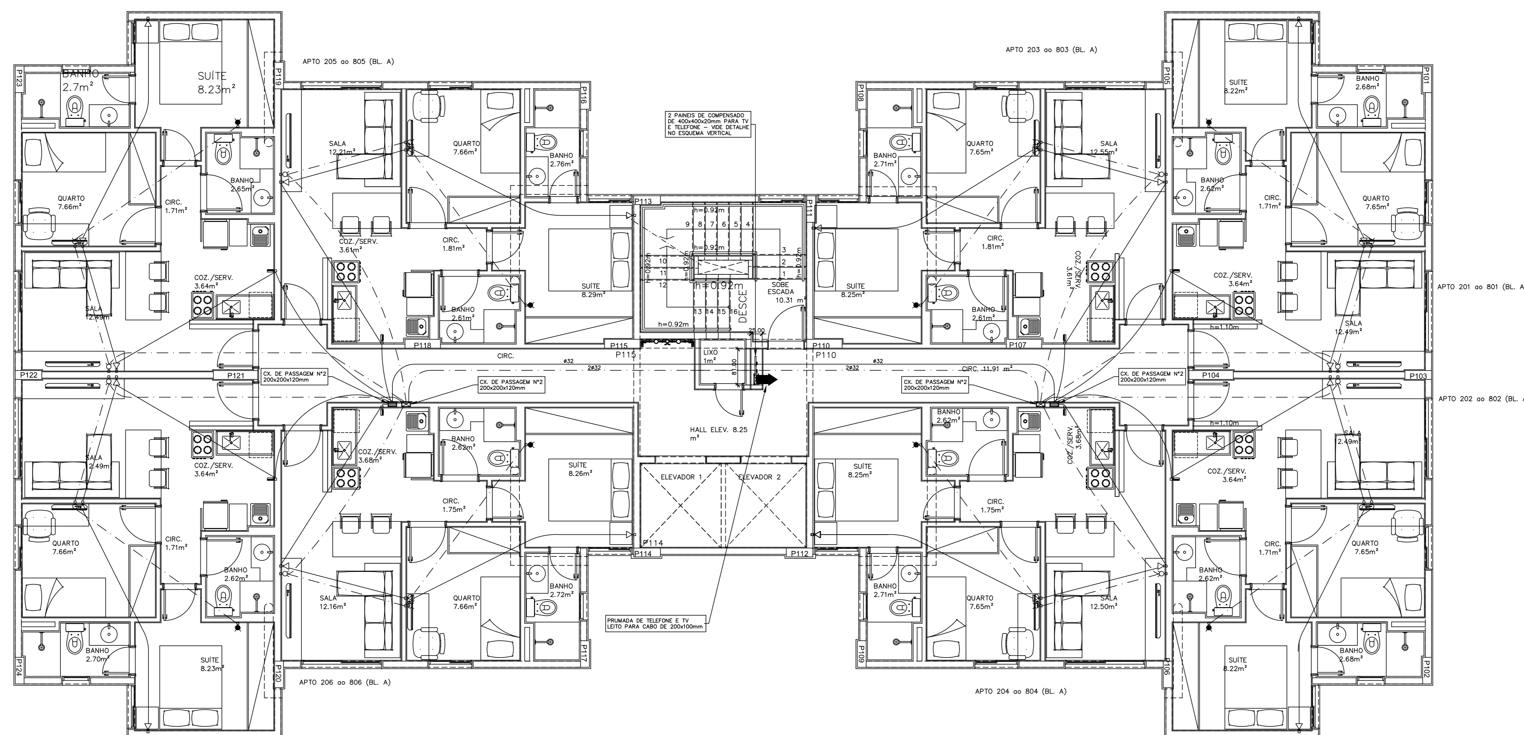
PLANTA BAIXA PAVIMENTO TIPO BLOCO A ESCALA 1:50
